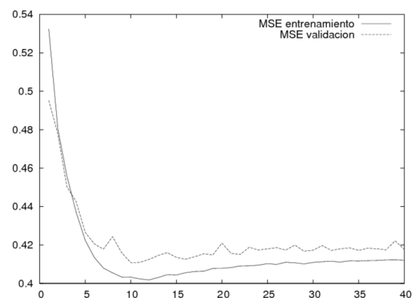
Figura 3. Detalle de la gráfica de la evolución del MSE durante el entrenamiento del modelo de 4-gramas. La mejor red fue encontrada en la época 10.
