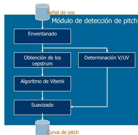
Figura 1. Diagrama de bloques del MDP.
