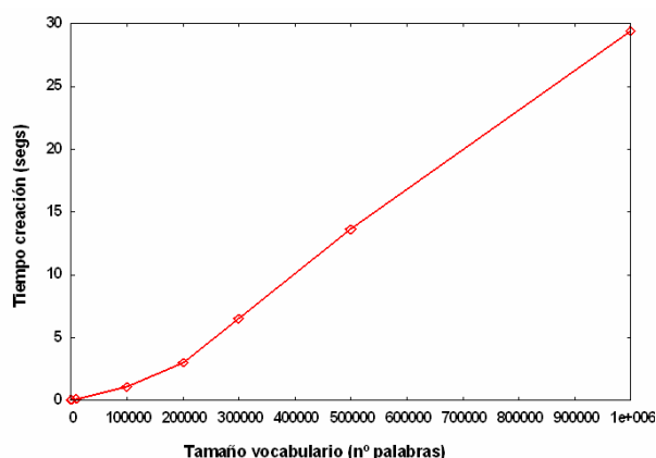
Figura 1. Latencia en el proceso de creación dinámica de gramáticas para RAH basadas en reglas.
