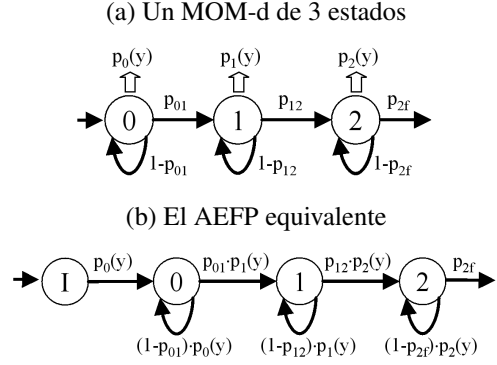
Figura 3. Cada transición en el MOM genera en el AEFN equivalente tantas transiciones como número de emisiones en el estado destino del MOM. El estado inicial adicional del modelo equivalente contiene transiciones a todos los estados iniciales del MOM.
