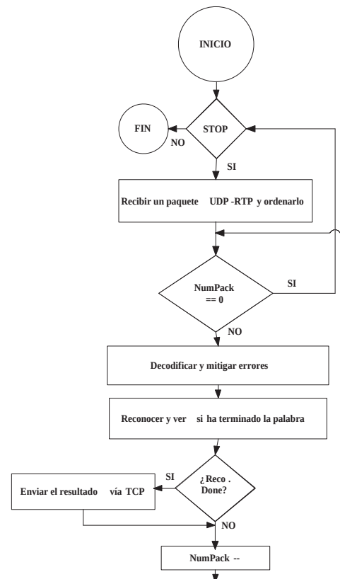
Figura 7. Organigrama del programa hijo del servidor UDP.
