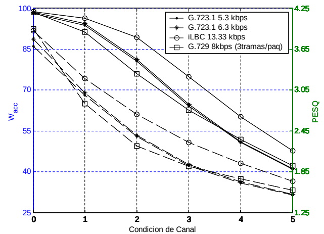
Figura 5. Comparativa de codificadores con empaquetado de 30 ms. El trazo continuo representa el W_{acc} (escala izquierda), mientras que el discontinuo se corresponde con el promedio PESQ ponderado (escala derecha).
