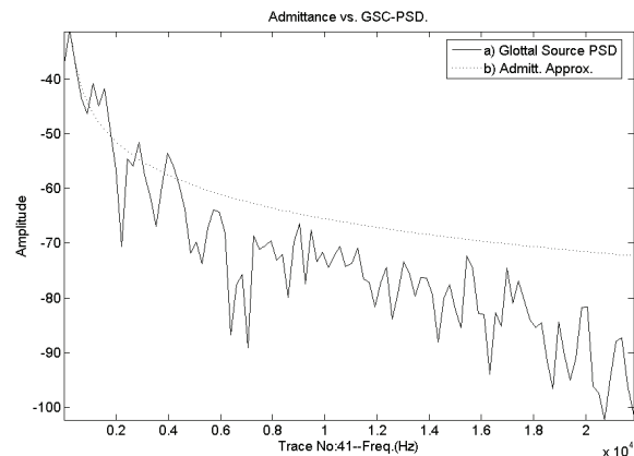
Figura 4. Ajuste de la admittance del modelo equivalente de 1 masa (línea de puntos) sobre la densidad espectral de potencia (en dB) de la componente dinámica de cubierta (línea continua) tras la última iteración para la estimación de la masa.
