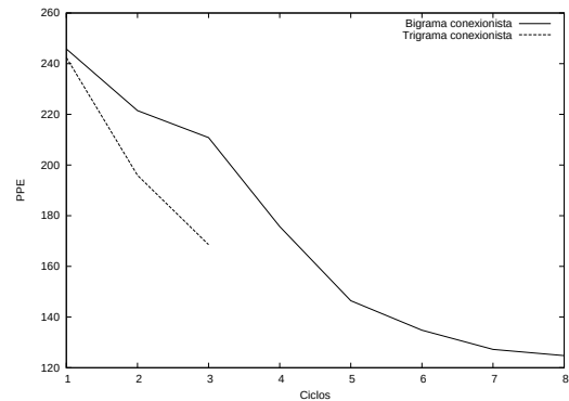
Figura 2. Evolución de la perplejidad de los modelos de lenguaje conexionistas (bigramas y trigramas) con codificación local para el corpus de palabras del Penn Treebank. Los trigramas conexionistas todavía no han llegado a la zona de convergencia, por lo que, con un mayor número de ciclos, se podría obtener un modelo de mayor precisión.
