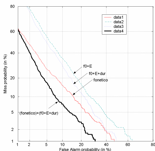
Figura 2. Resultados para el sistema basado en el modelado de lenguaje de segmentos prosódicos
