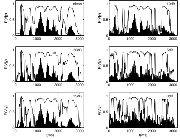
Figura 1. Probabilidad P(V|y) de que el frame y sea voz para cada frame de una frase, evaluada a diferentes SNRs. La amplitud de la señal (para valores positivos) también se ha representado en cada gráfica.
