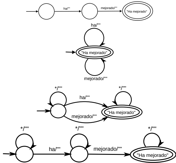
Figura 3. Modelos de lenguaje representados por autómatas de estado finito (los cuales son también transductores) que modelan la frase “ha mejorado”. De arriba hacia abajo: el primero acepta solo la frase “ha mejorado”; el segundo acepta una secuencia de las palabras “ha” y/o “mejorado” en cualquier orden y número de repeticiones; el tercero acepta una secuencia de fonemas cualquiera (representado por el *) + “ha” o “mejorado” + secuencia cualquiera de fonemas; finalmente el último modelo acepta una secuencia de fonemas cualquiera + “ha” + secuencia de fonemas cualquiera + “mejorado” + secuencia de fonemas cualquiera.
