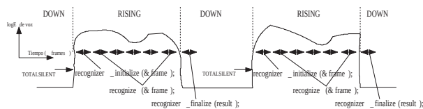
Figura 9. VAD del servidor.
