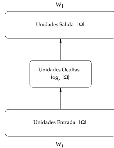
Figura 1. Perceptrón Multicapa para obtener una codificación distribuida subsimbólica a partir de la representación local de los datos. La entrada y salida son codificaciones locales de la palabra. Mediante el entrenamiento de la red podemos conseguir una codificación distribuida en la capa oculta.
