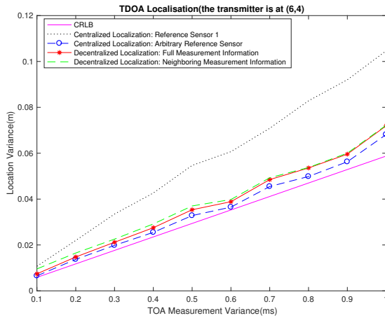
Fig. 1. TDOA Localisation
