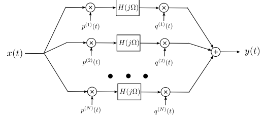
Fig. 1. N-path filter.
