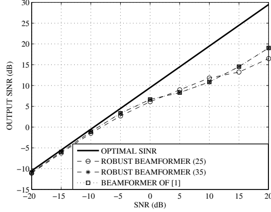
Fig. 1. Output SINR versus SNR. INR = 20 dB, K = 100 .
