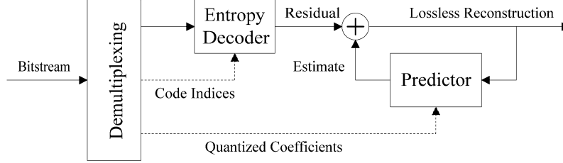
Fig. 2. MPEG-4 ALS decoder
