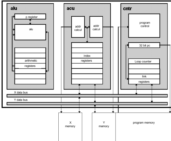
Fig. 1. Gepard DSP architecture, ©AMS Austria Mikrosysteme International AG
