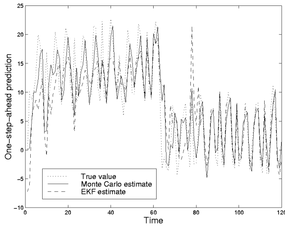
Figure 4: Actual output data [...], Monte Carlo posterior mean estimate using 50 samples [—] and EKF estimate [- -].
