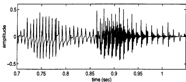
(d) Synthesised speech, pitch 0.75 \times f_0
