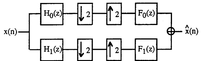
Fig. 1. 2 Band QMF Filterbank
